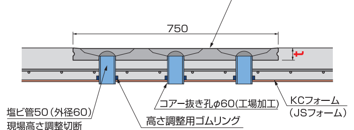
■A-A'断面図
