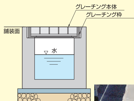
■A-A'断面図
