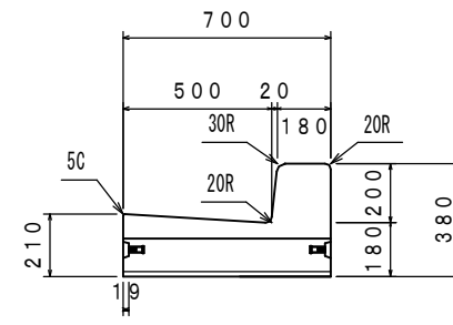
L型エプロンC型両R 斜H50 右
