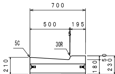
L型エプロンC型両R 斜H50 左
