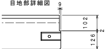
目地部詳細図
