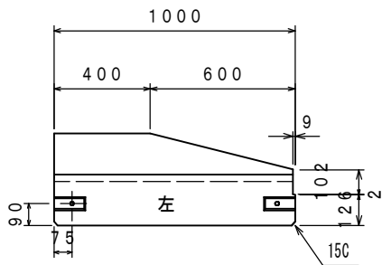
L型エプロンC型両R 斜H50 左
