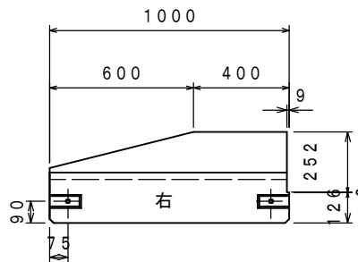
L型エプロンC型両R 斜H50 右
