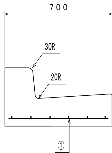
目地部詳細図
