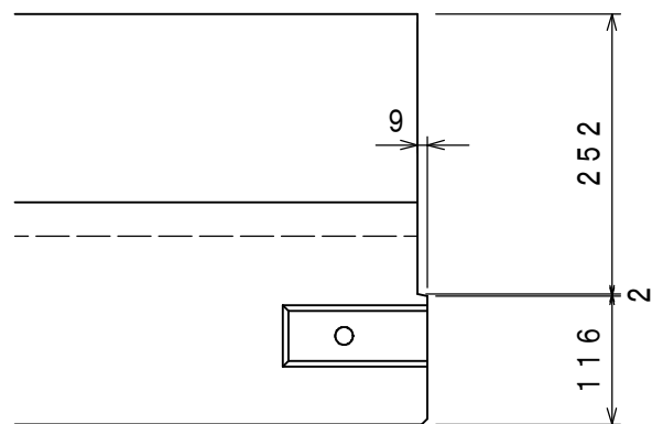
目地部詳細図
