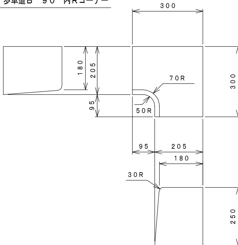
歩車道B 90° 内Rコーナー
