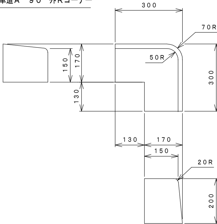
歩車道A 90° 外Rコーナー
