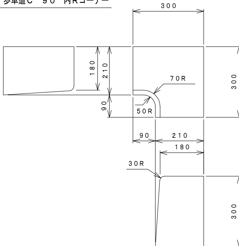
歩車道C 90° 内Rコーナー
