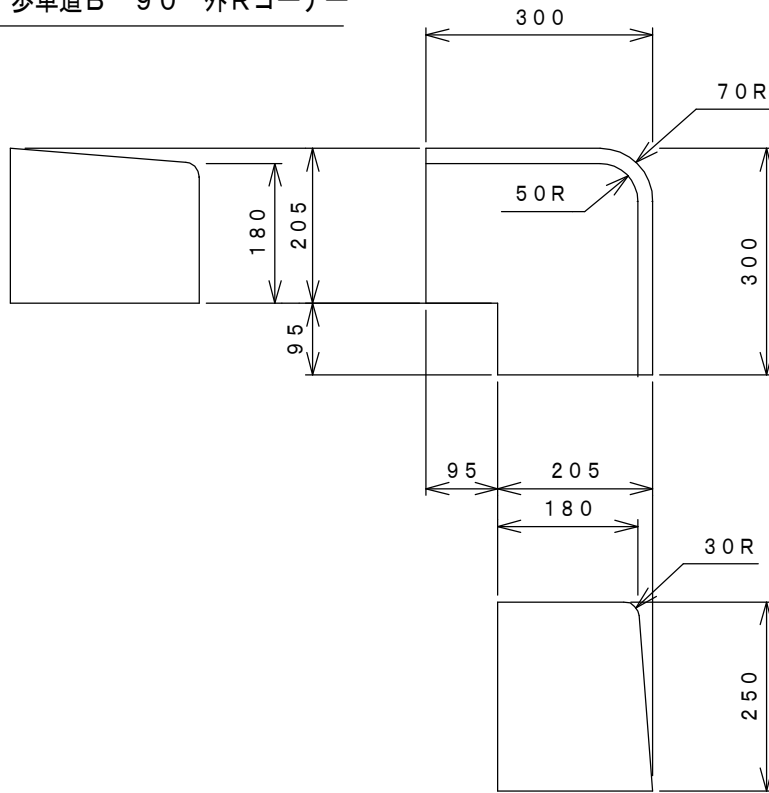
歩車道B 90° 外Rコーナー
