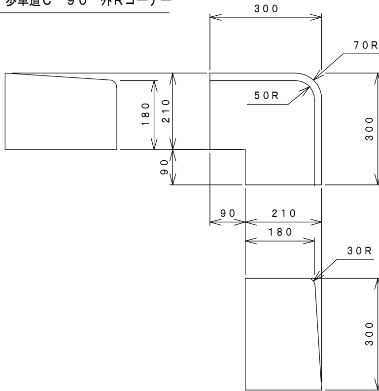
歩車道C 90° 外Rコーナー
