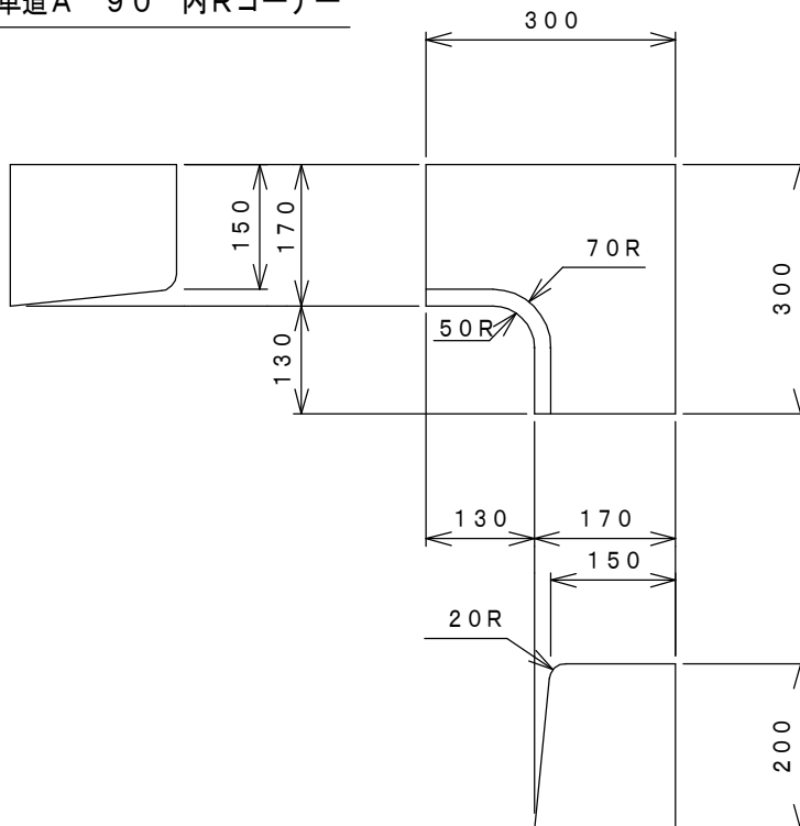
歩車道A 90° 内Rコーナー
