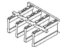
スベリ止め詳細図
