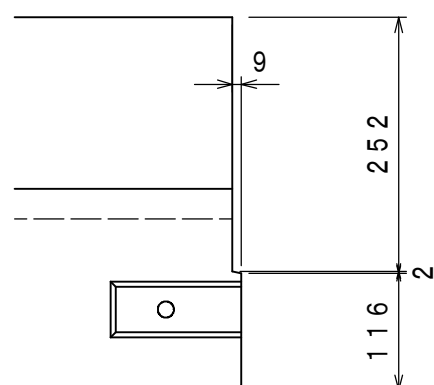
目地部詳細図
